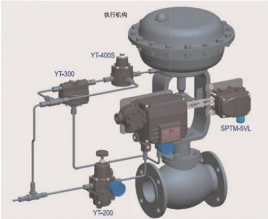
YT-400S YT-420S YT-430S 单作用安装图例
