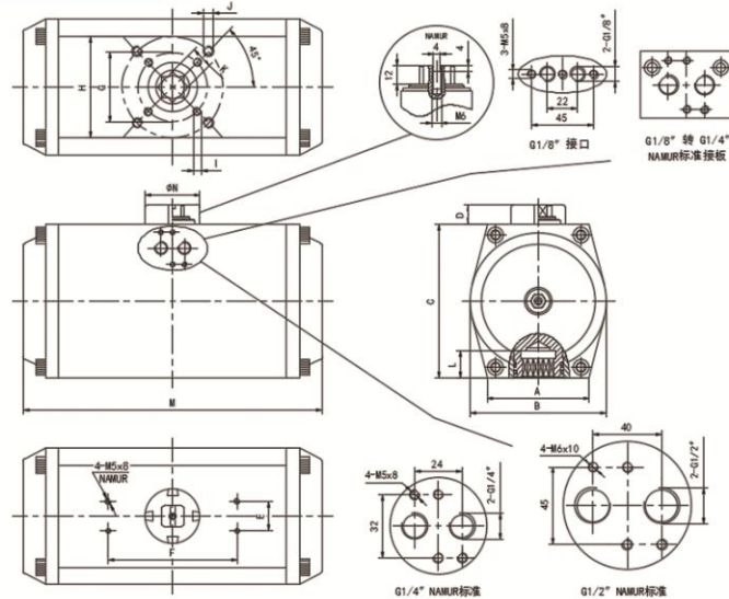
GT系列执行器安装尺寸表 GT series actuator dimension table
