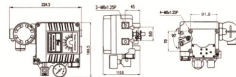
▲角行程
